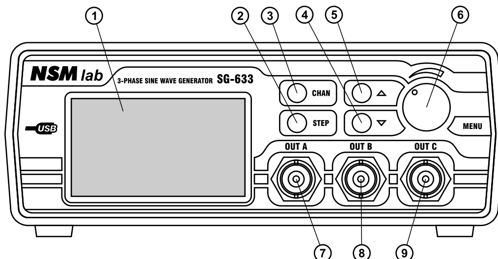
Рис. 1. Внешний вид передней панели генератора SG-633.
